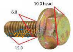
M6 8.8 Flange Bolts 25pcs
